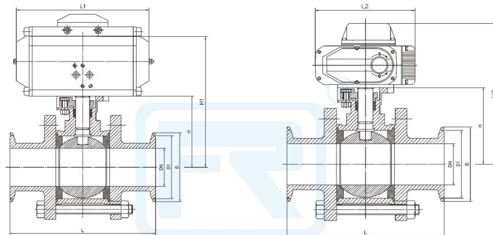
主要外形尺寸表 Main dimensions table
