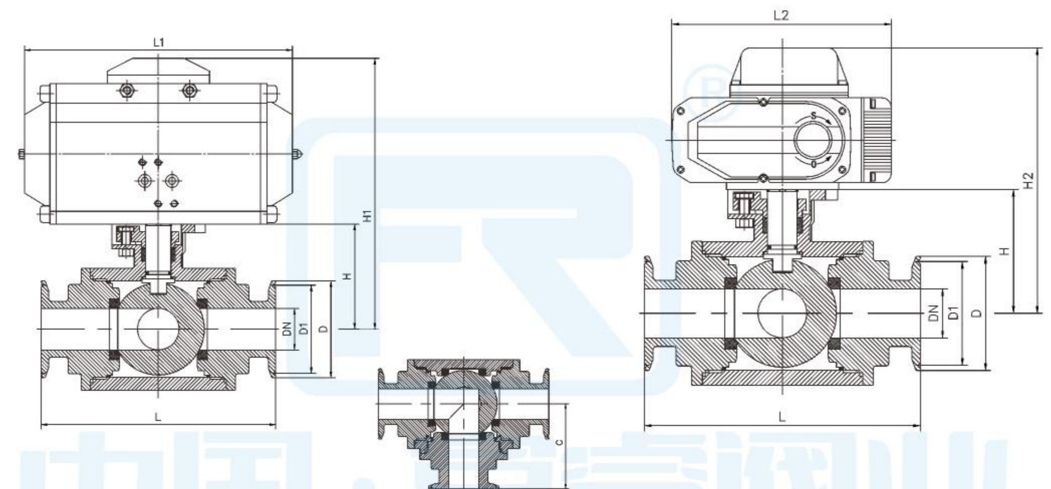
主要外形尺寸表 Main dimensions table
