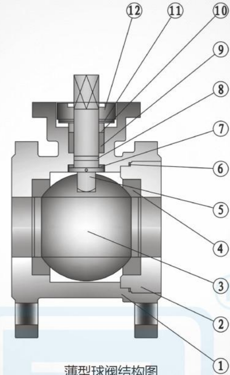
薄型球阀结构图
