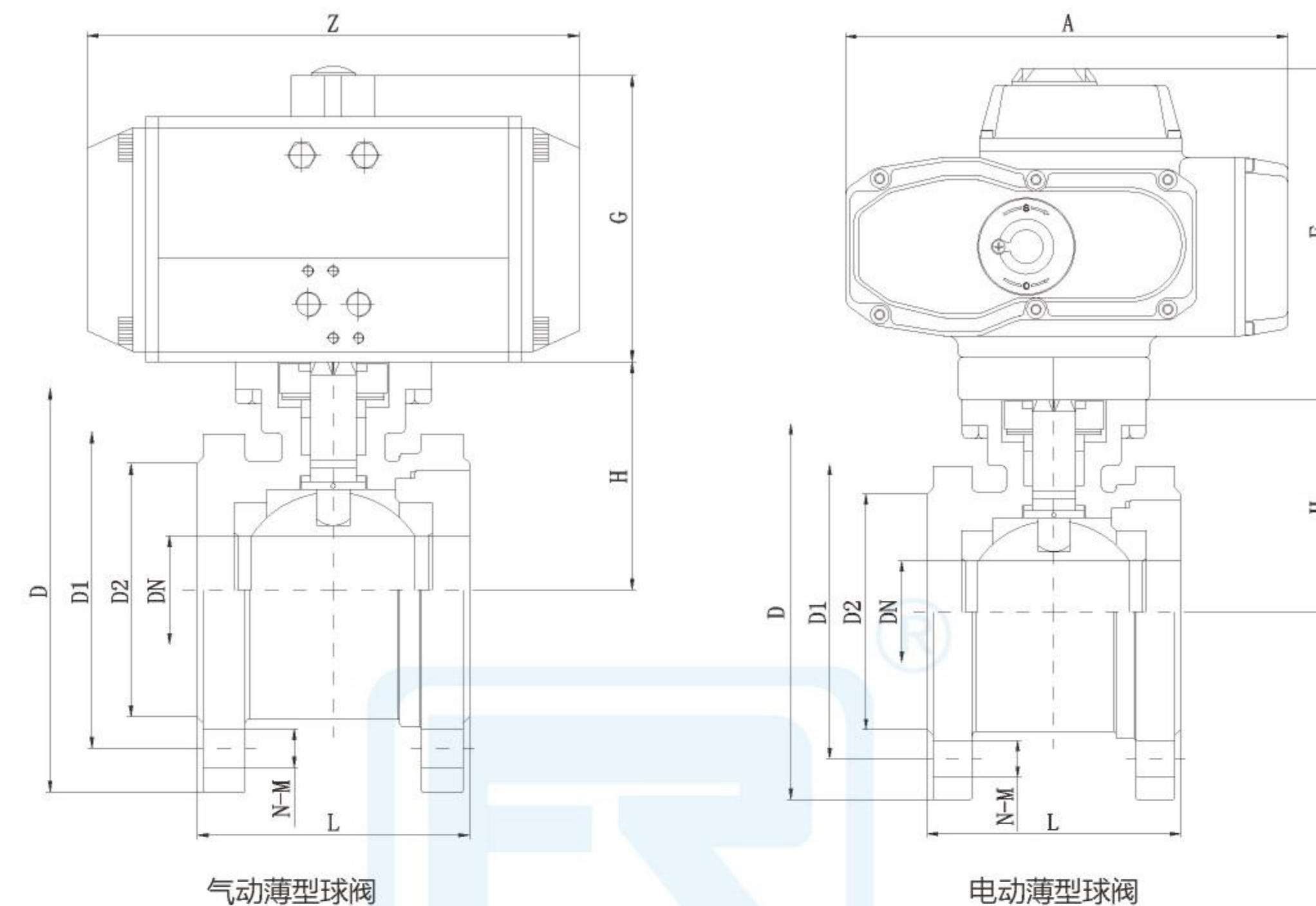
ASME CLASS150 主要外形尺寸表 Main dimensions table
